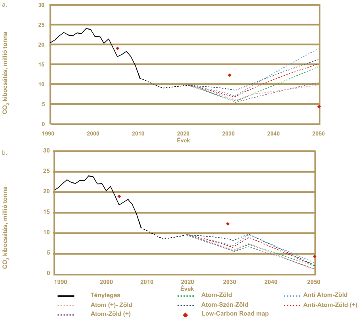
2. ábra: Villamos energia és kapcsolt hőtermelés CO 2 kibocsátása CCS nélkül (a.) és CSS-sel (b.)
