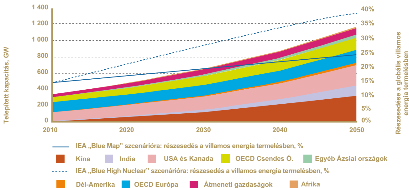
32. ábra. A nukleáris „reneszánsz” forgatókönyv: az atomenergia arányának gyors növekedése a globális villamosenergia-termelésben 2050-ig Forrás: IEA, NEA
